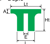
Perfil "T" Duplo
