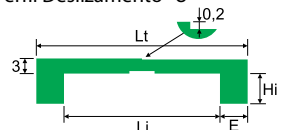
Perfil Deslizamento "U"
