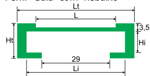
Perfil Deslizamento "U"
