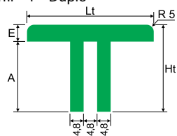
Perfil "T" Duplo
